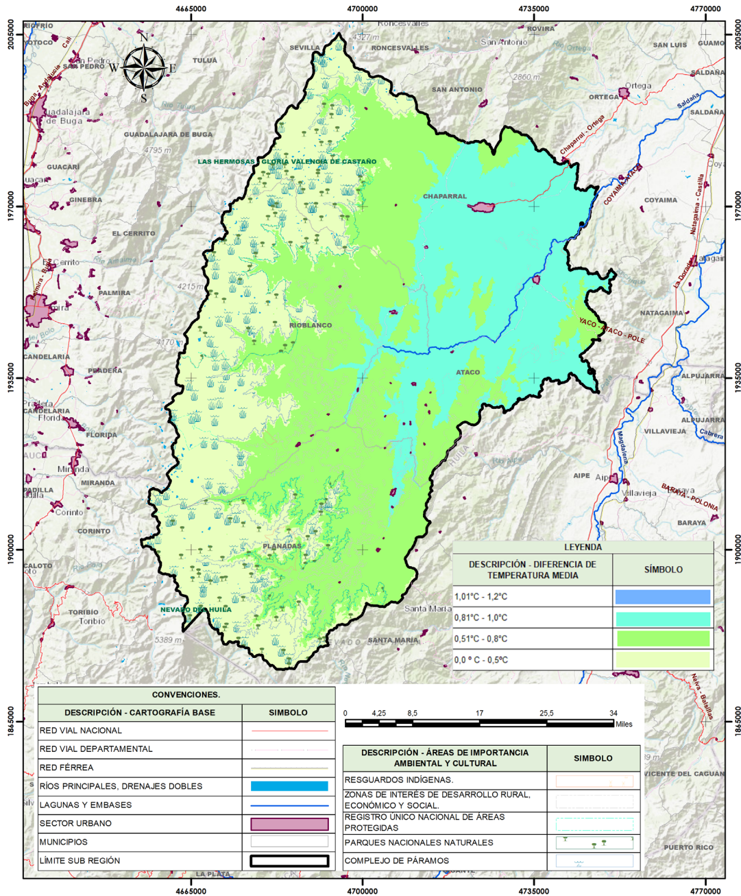
Ilustración 3. Escenario RPC 6.0 de cambio climático para 2040 para la precipitación promedio y la temperatura media para la subregión PDET Sur de Tolima
